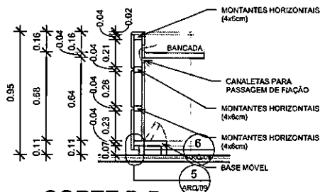
4 CORTE B-B 1:20
