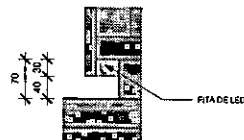
6 DET. FITA DE LED M. 03B 1:5
