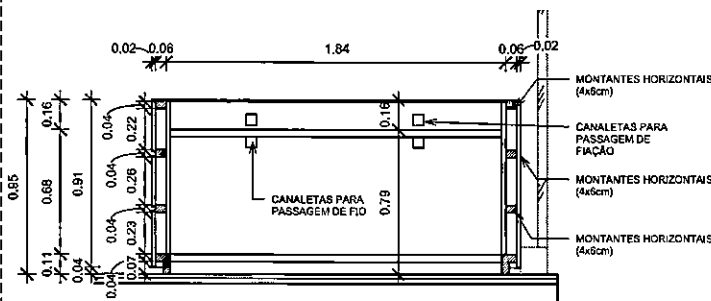
4 CORTE B-B MÓDULO 02B 1:20
