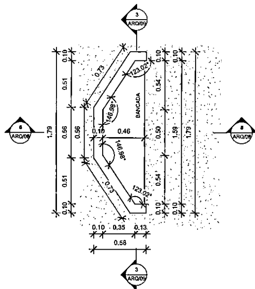
1 DET. BANCADA 1:20
