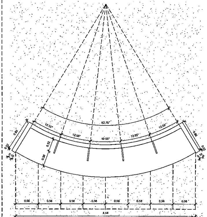
1 MÓDULO 03B 1:20
