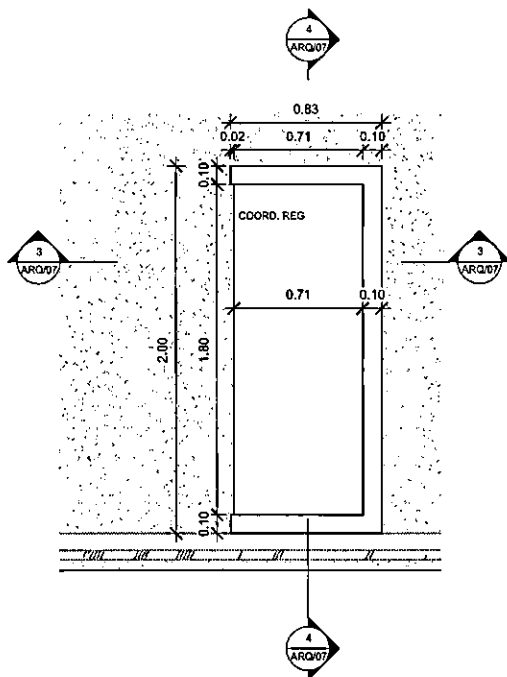
1 MÓDULO 02B 1:20
