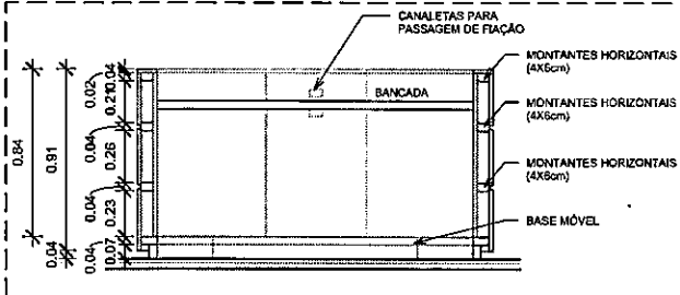
3 CORTE A-A 1:20
