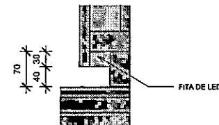
5 DET. FITA DE LED M. 02B 1:5
