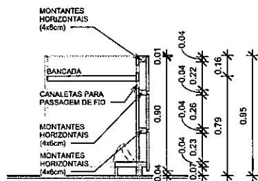
3 CORTE A-A MÓDULO 02B 1:20
