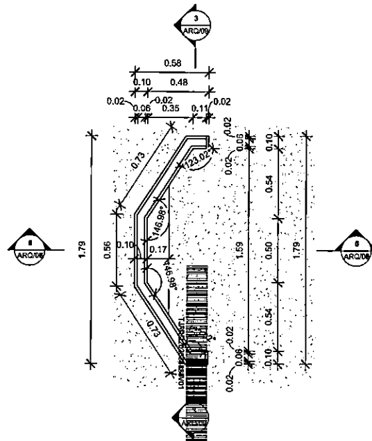
2 P.B. BANCADA 1:20
