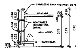
3 CORTE A-A MÓDULO 03B 1:20
