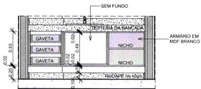
2 VISTA INTERNA SANIT.02 1 : 25
