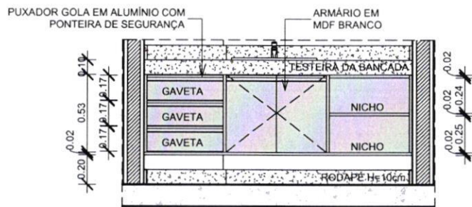
1 VISTA EXTERNA SANIT.02 1 : 25
