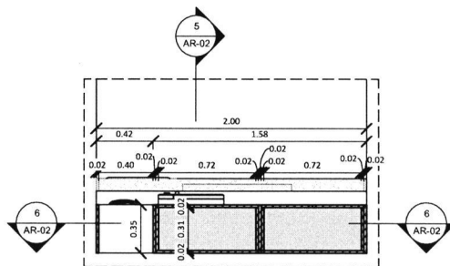
1 ARMÁRIO ALTO 1 : 25
