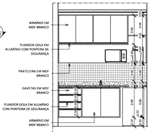
4 VISTA EXTERNA. 1 : 25
