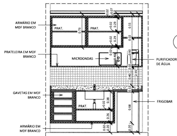
6 VISTA INTERNA. 1 : 25
