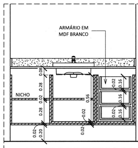
5 Corte 8 1 : 20
