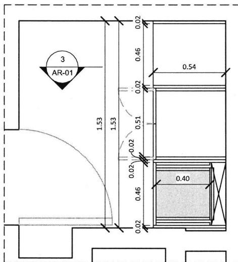
1 ARMÁRIO - SANITÁRIO 1 : 20
