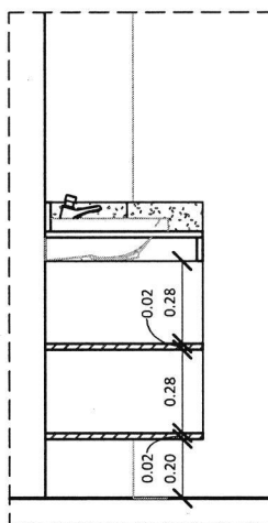
3 Corte 6 1 : 20
