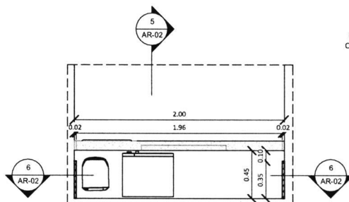
2 ARMÁRIO MÉDIO 1 : 25
