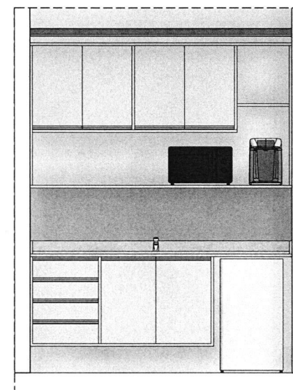
7 VISTA FRONTAL. 1 : 20
