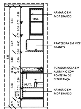
5 Corte 5 1 : 25
