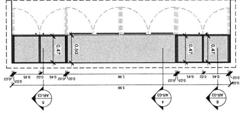
PLANTA BAIXA 1 : 25
