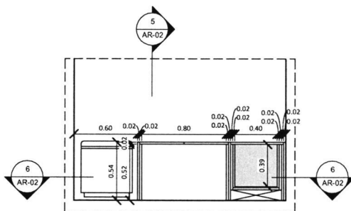
3 ARMÁRIO BAIXO 1 : 25
