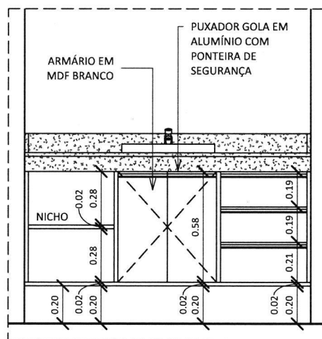
2 VISTA EXTERNA 1 : 20
